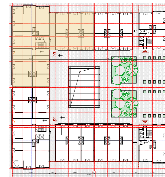
OSNOVA VI SPRATA R=1:150
